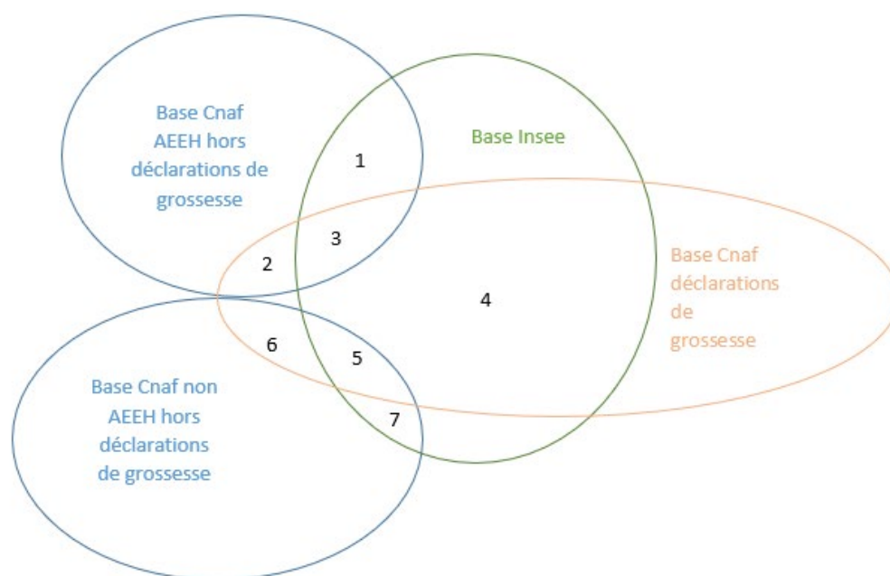
Graphique 2 Schéma d'identification des liens entre bases de sondage
